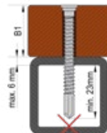
Anwendungsbeispiel Holz auf Stahl
